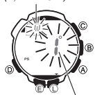
Угловая величина магнитного склонения
